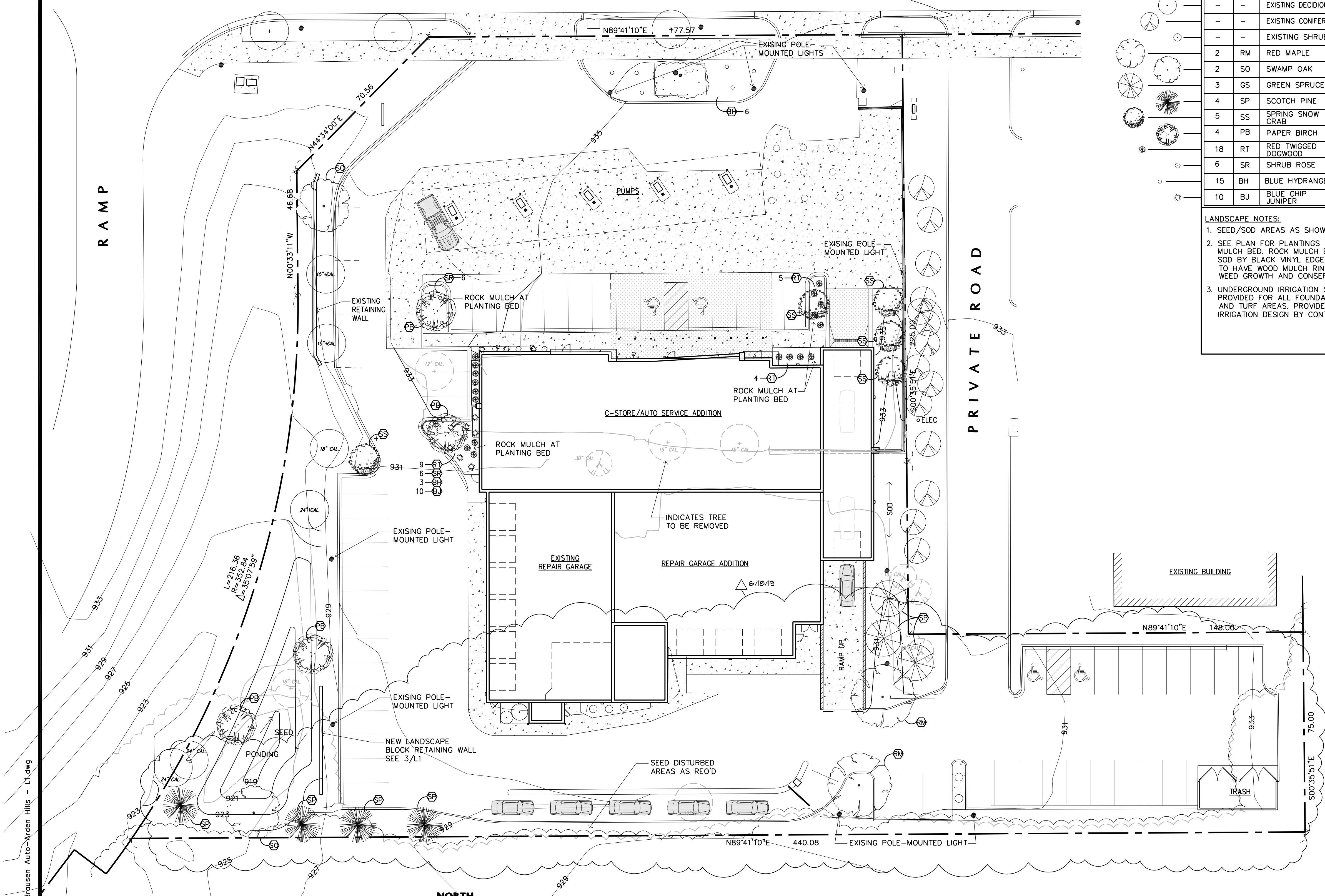
1 LANDSCAPE L1 SCALE: 1" = 20'-0"
